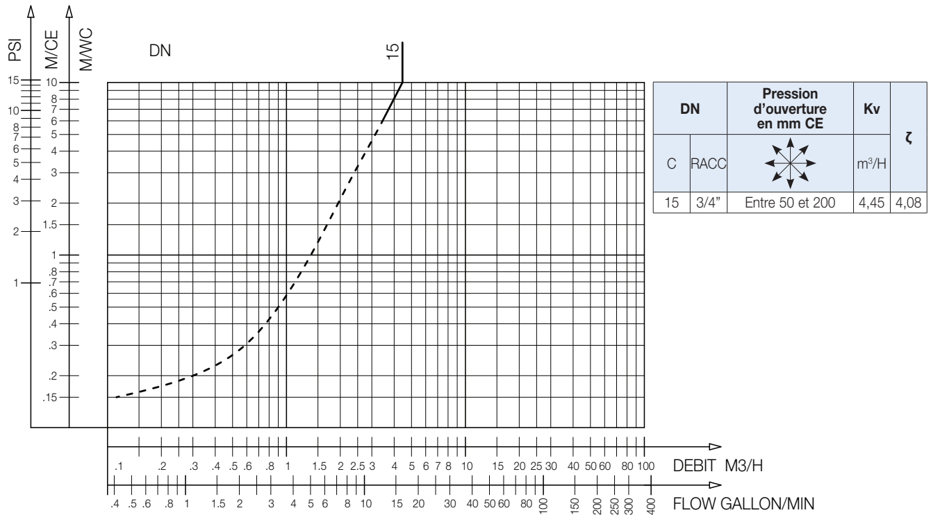
WF Compact Abaque des pertes de charge
