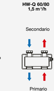
HW-Q60/80: Collegamento da destra
