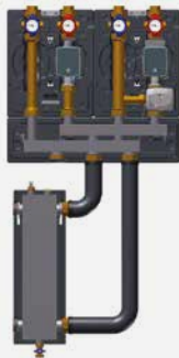
HW80/120: Collegamento da sinistra
