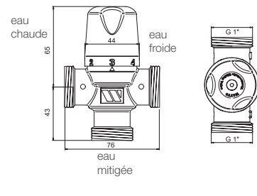
Filetage mâle 1"
