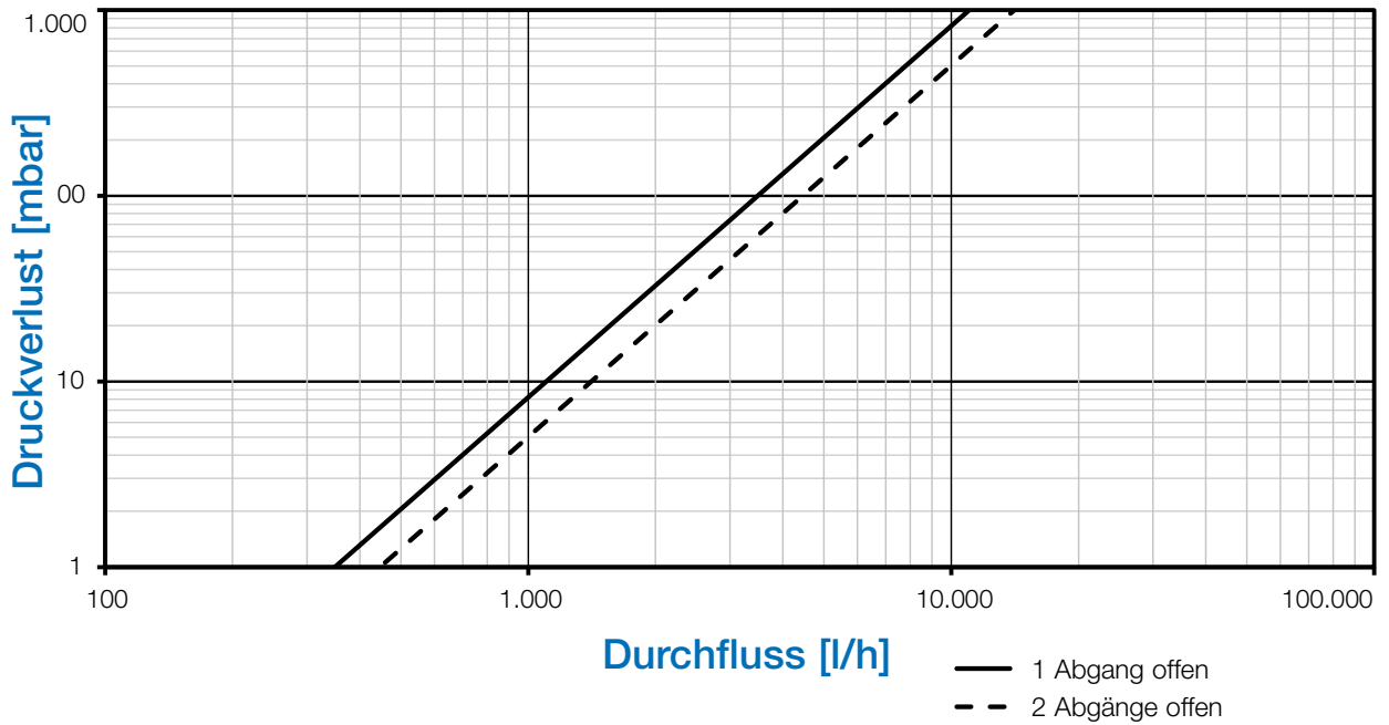
Druckverlustdiagramm VB20-2
